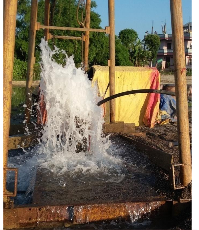
डिप वोरिङ्ग सम्पन्न भई कम्प्रेसर लगाईदै
