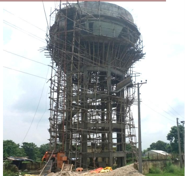
प्रेमवस्ती कालिका खानेपानी आयोजनाको सम्झौता देखी निर्माण सम्पन्न हन लागेको टंकीको दृश्यहरु
